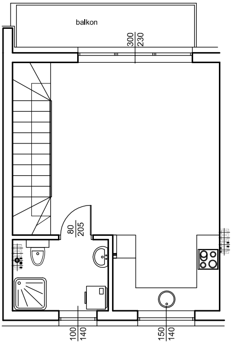
ZESTAWIENIE POWIERZCHNI UŻYTKOWEJ PIĘTRO
